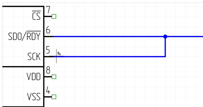
Рис. 57 Проложенный проводник
