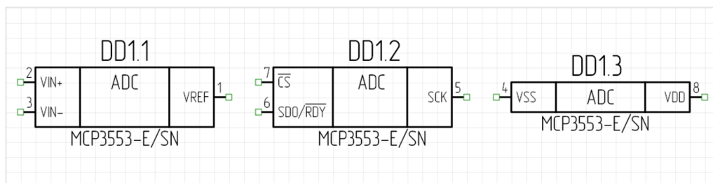
Рис. 31 Размещение многосекционного компонента
