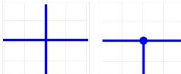
Рис. 62 Пересечение и объединение цепей на схеме
