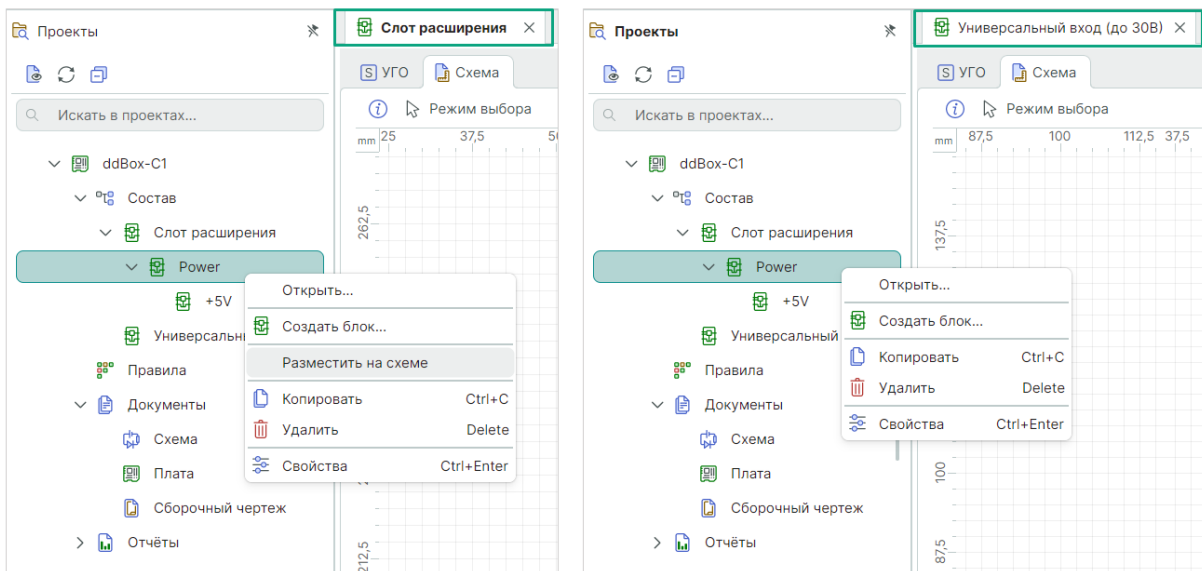
Размещение блока нижнего уровня на «родительской» схеме допустимо
