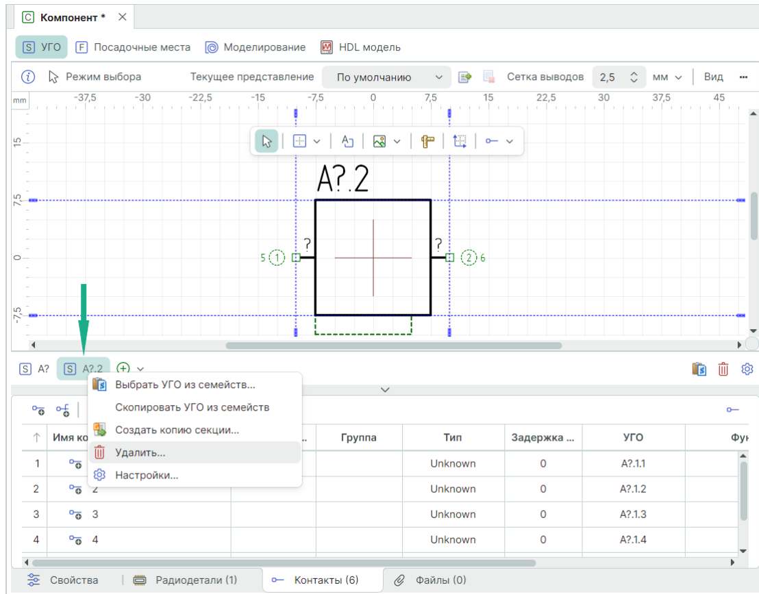
Рис. 215 Удаление секции
