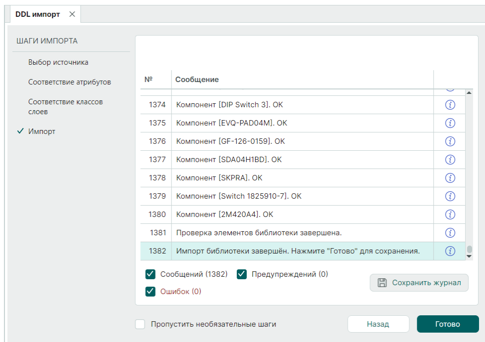
Рис. 28 Импорт библиотеки
