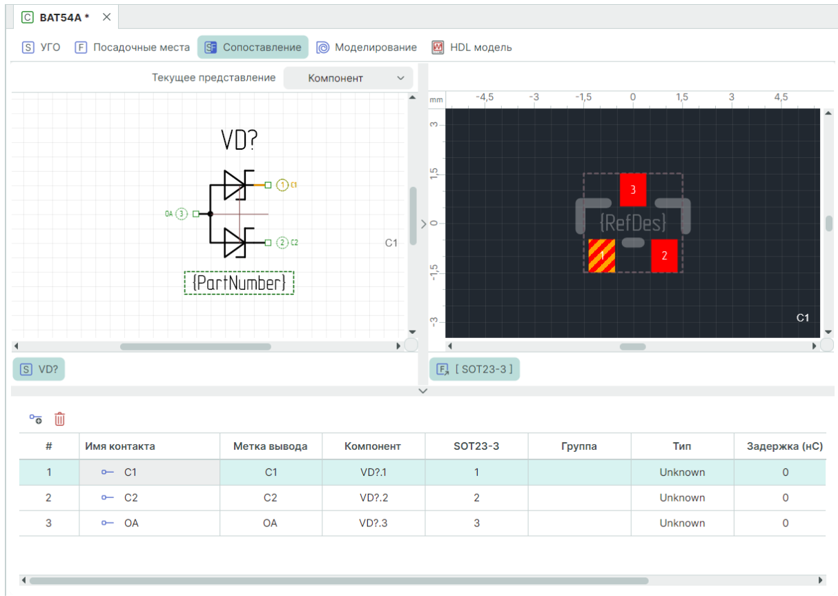
Рис. 253 Вкладка «Сопоставление»
