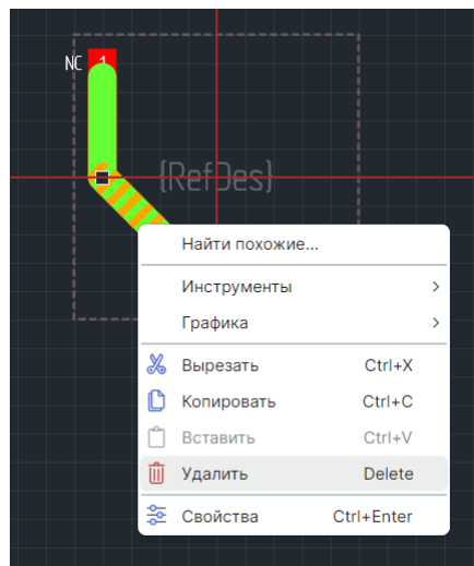
Рис. 129 Удаление сегмента
