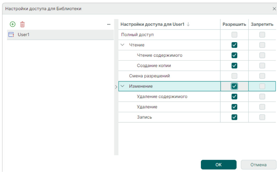
Рис. 78 Настройка разрешений для пользователя
