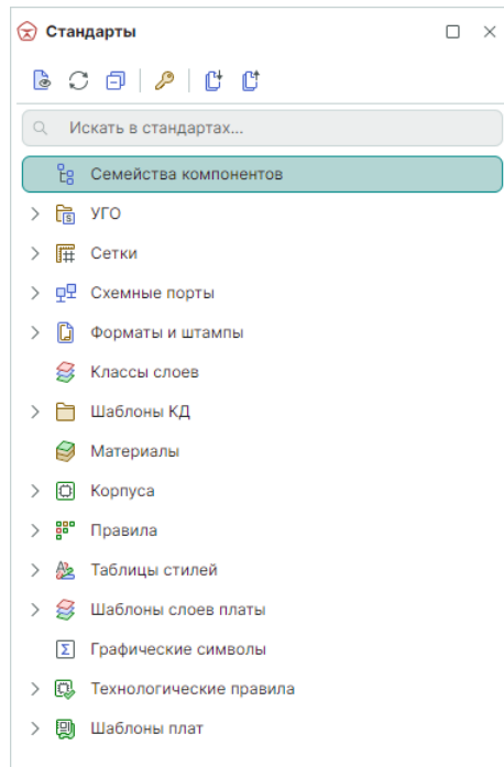
Рис. 80 Панель «Стандарты»
