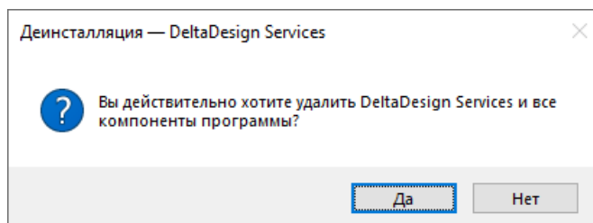
Рис. 41 Подтверждение удаления
