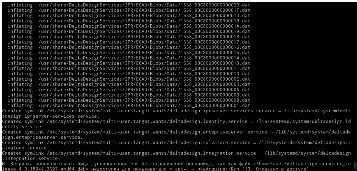
Рис. 37 Завершение установки
