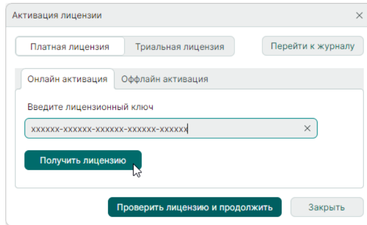
Рис. 44 Получение лицензии
