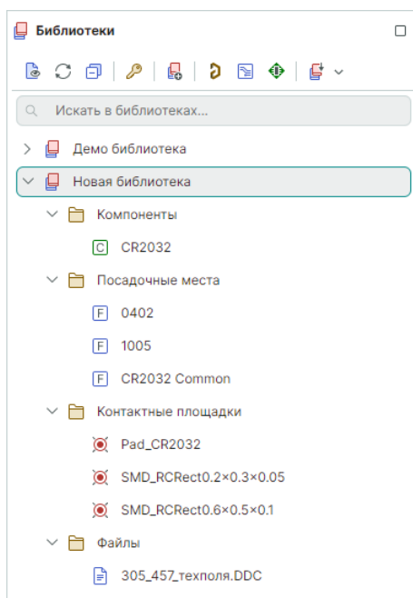
Рис. 81 Панель «Библиотеки»
