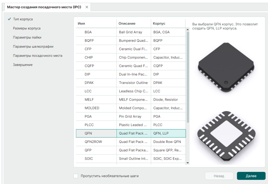
Рис. 148 Выбор корпуса для создания посадочного места
