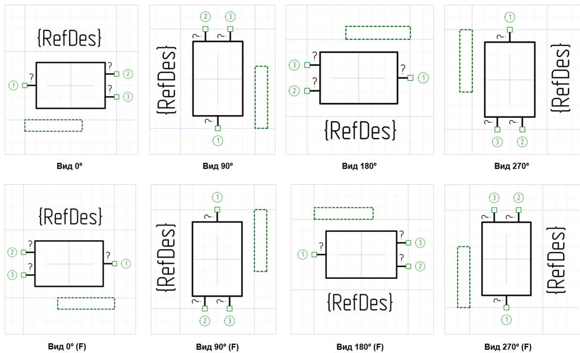
Рис. 185 Варианты ориентации УГО
