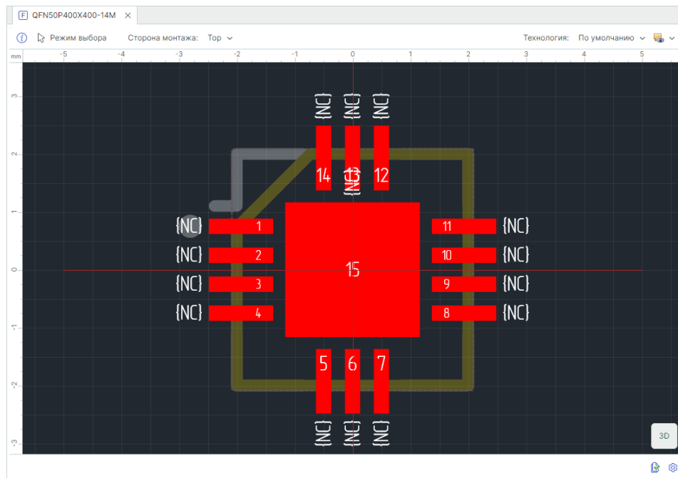
Рис. 156 Созданное посадочное место
