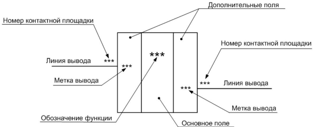
Рис. 225 Типовое УГО элемента цифровой техники
