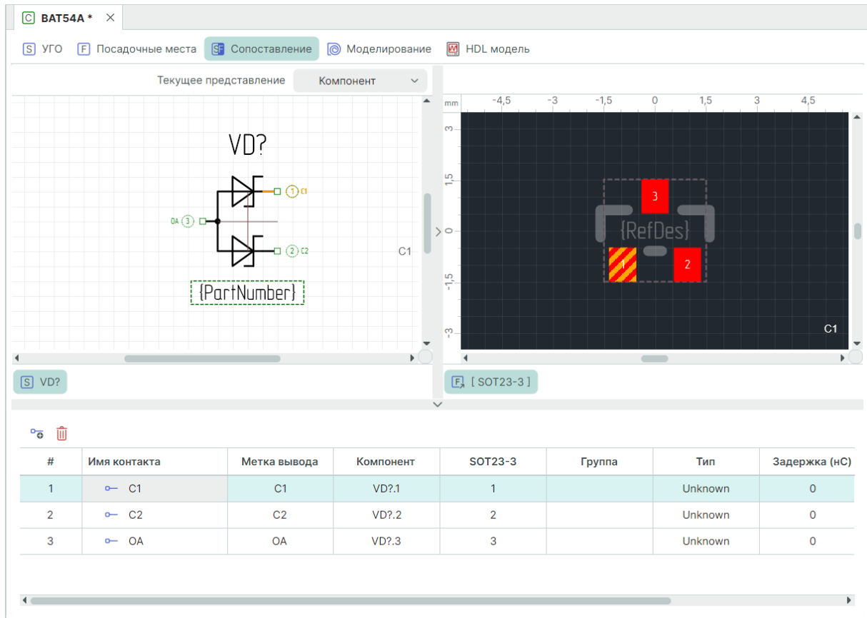
Рис. 253 Вкладка «Сопоставление»
