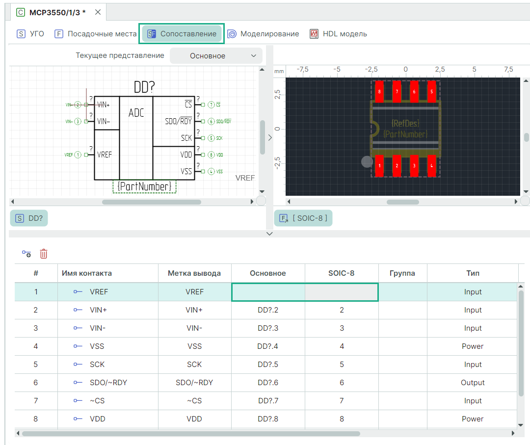
Рис. 273 Вкладка «Сопоставление»
