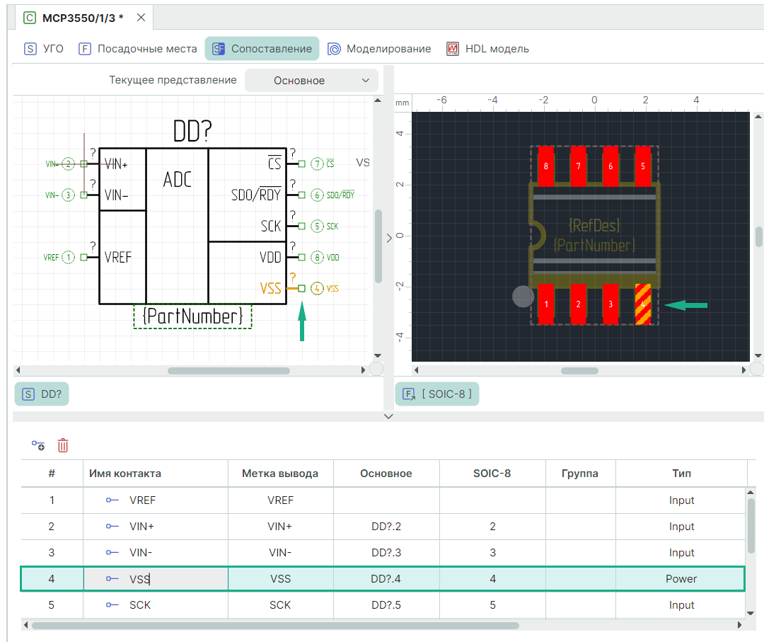
Рис. 274 Сопоставленные выводы и контактные площадки
