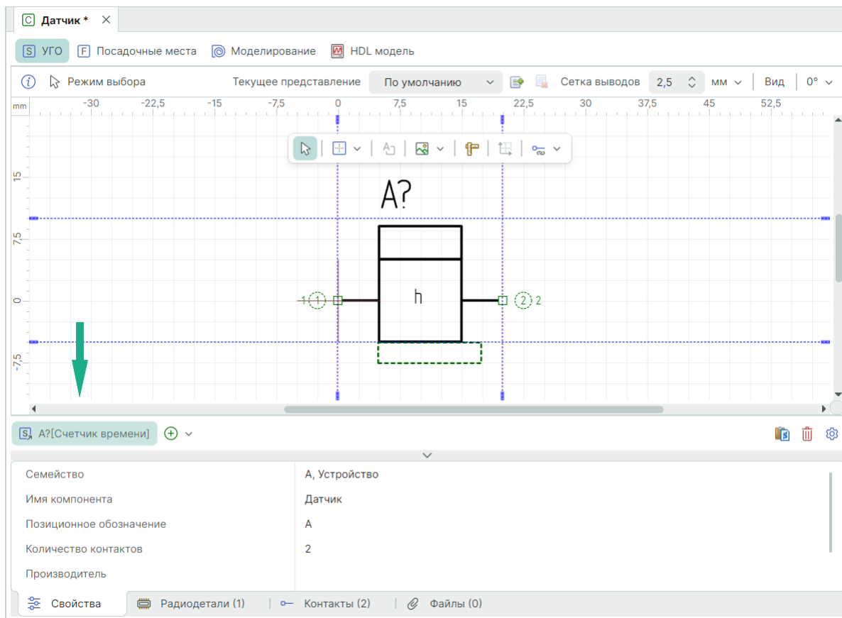
Рис. 203 Отображение имени выбранного из Стандартов УГО
