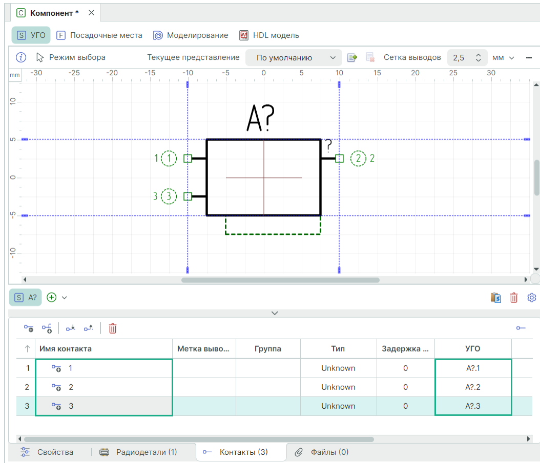
Рис. 237 Размещенный вывод сопоставлен с контактом
