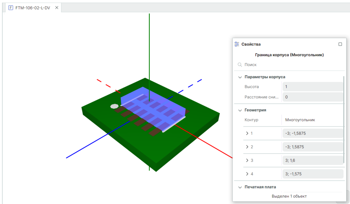
Рис. 158 3D-модель компонента
