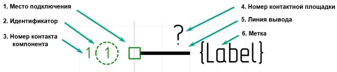
Рис. 171 Составляющие вывода
