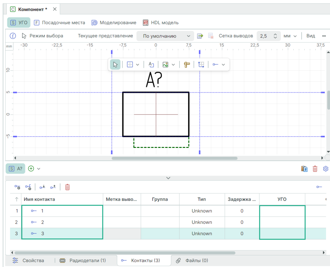
Рис. 234 Контакты, не сопоставленные с выводами УГО
