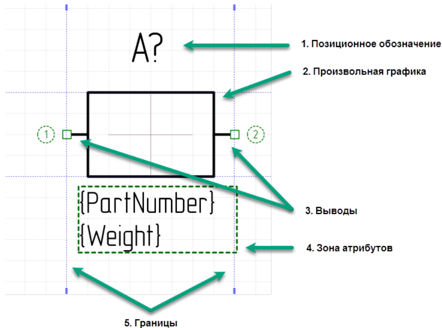
Рис. 170 Структурные элементы УГО
