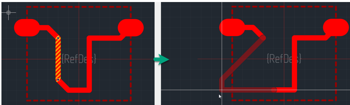
Рис. 128 Перемещение характерной точки трека
