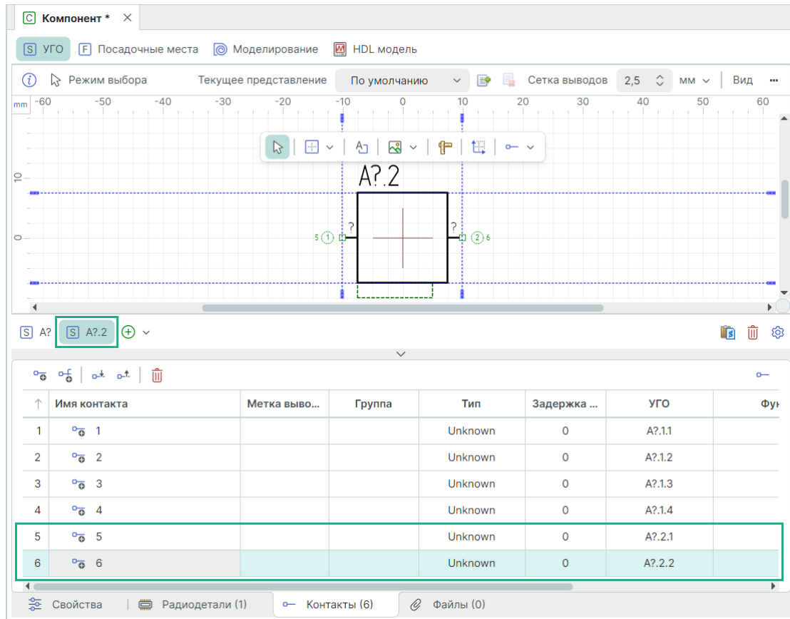
Рис. 214 Новая секция
