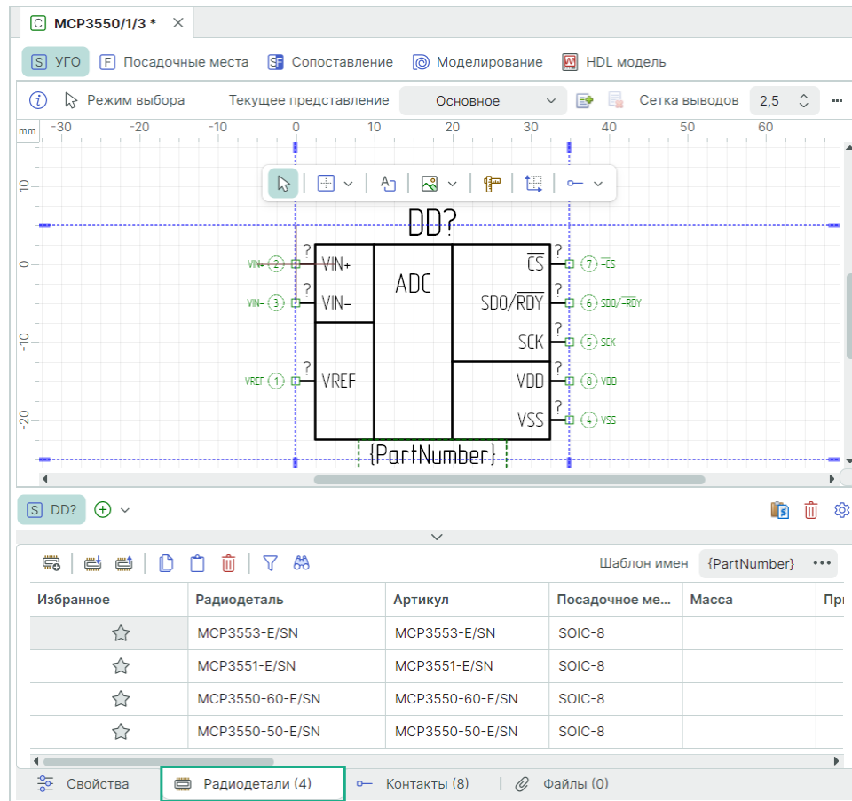
Рис. 303 Вкладка «Радиодетали»
