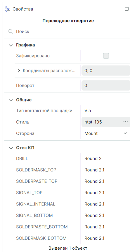
Рис. 130 Свойства переходного отверстия
