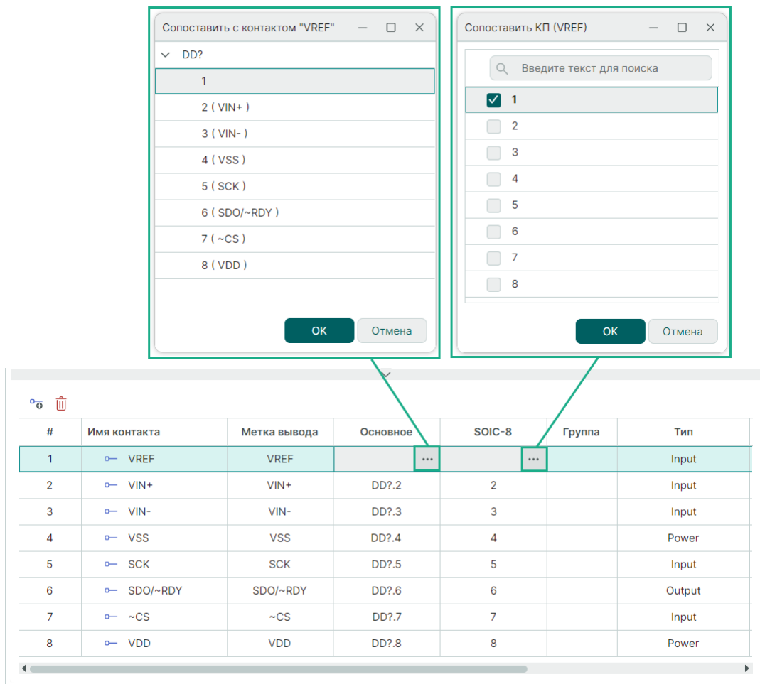
Рис. 277 Выпадающие меню с выводами и КП в таблице контактов для
