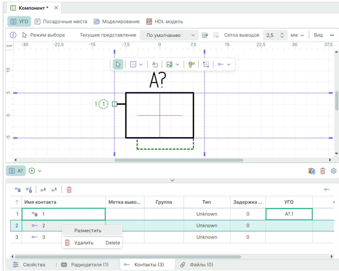
Рис. 235 Размещение выводов на основе контактов
