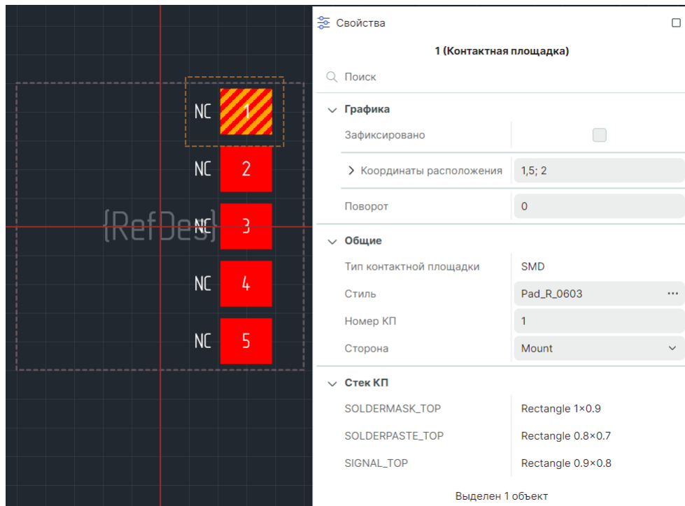
Рис. 117 Свойства контактной площадки
