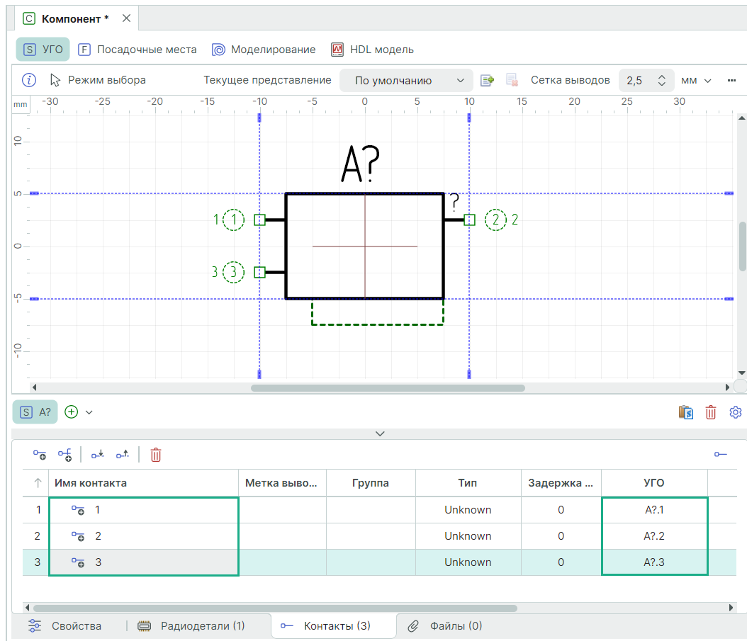
Рис. 228 Размещенный вывод сопоставлен с контактом
