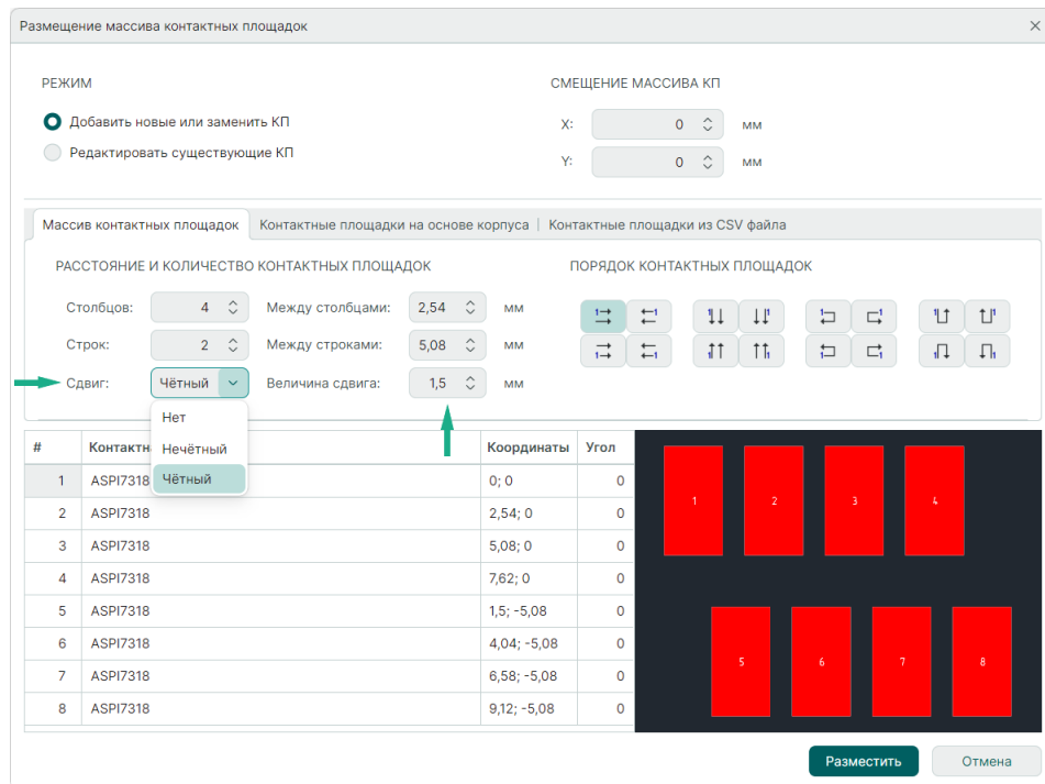
Рис. 91 Установка сдвига для контактных площадок
