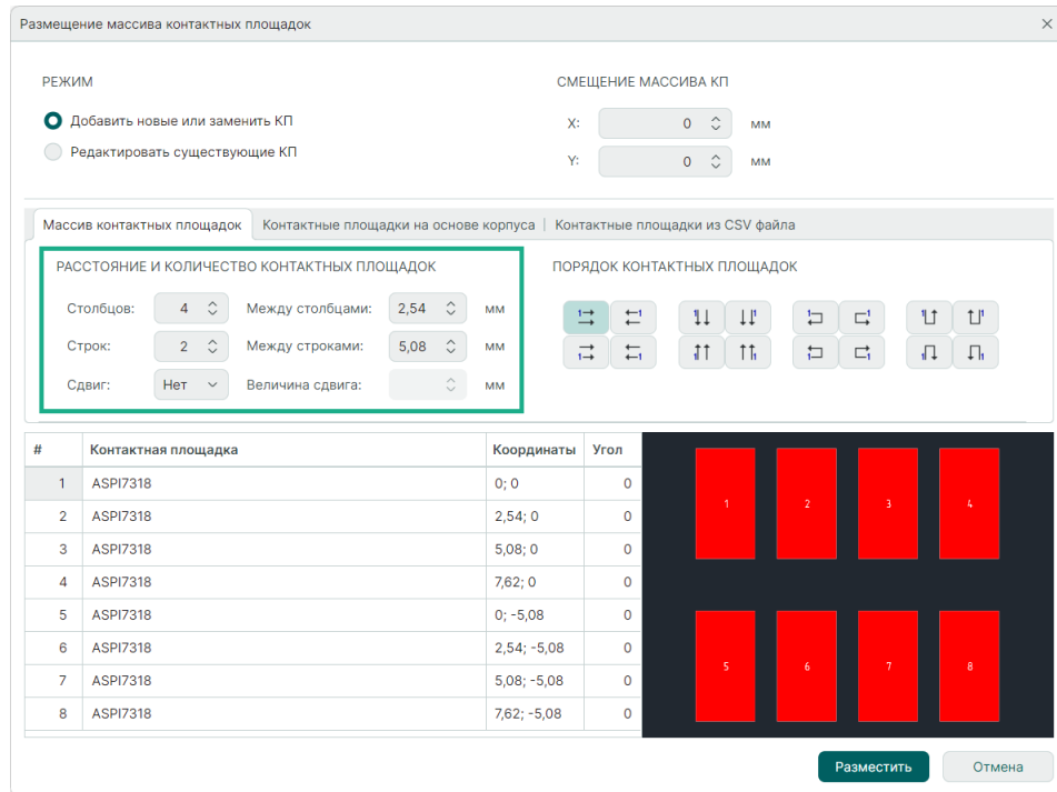
Рис. 90 Геометрические параметры массива контактных площадок
