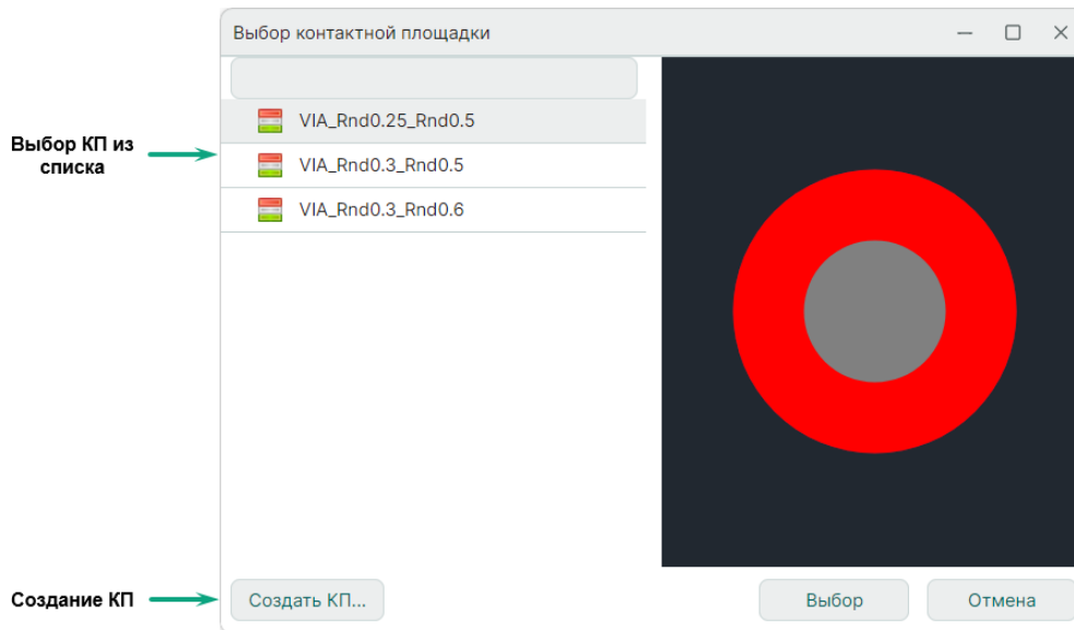
Рис. 106 Выбор типа размещаемого переходного отверстия
