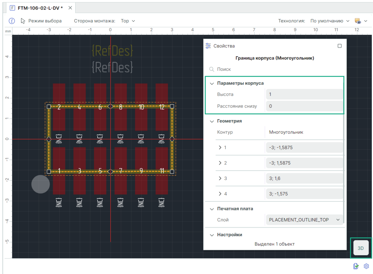
Рис. 148 Создание 3D-модели посадочного места
