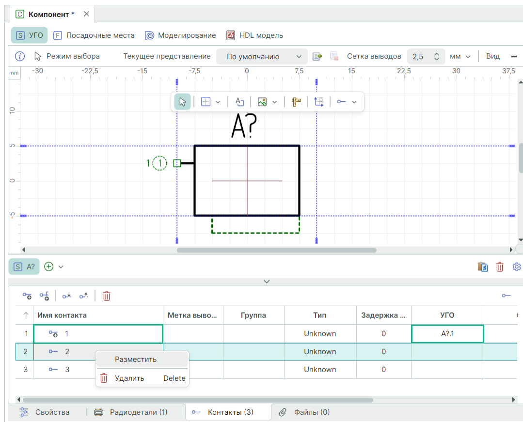
Рис. 226 Размещение выводов на основе контактов
