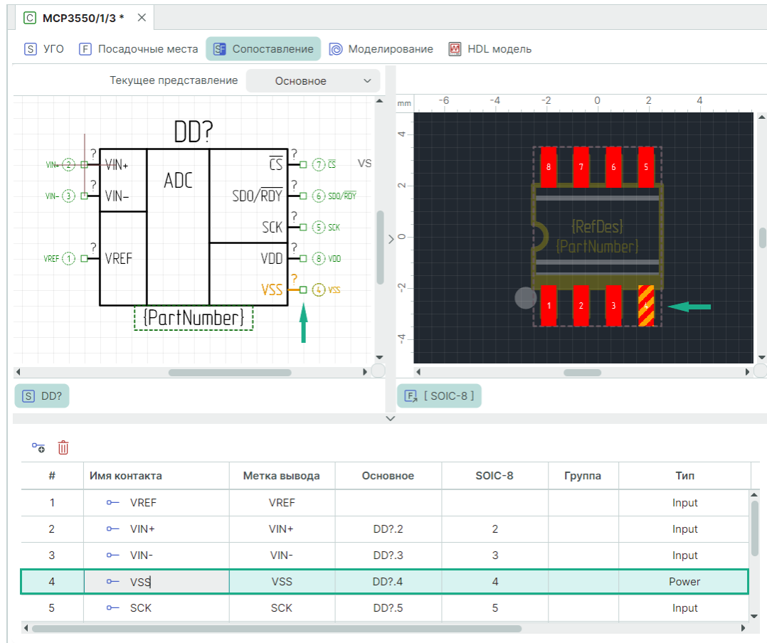
Рис. 265 Сопоставленные выводы и контактные площадки
