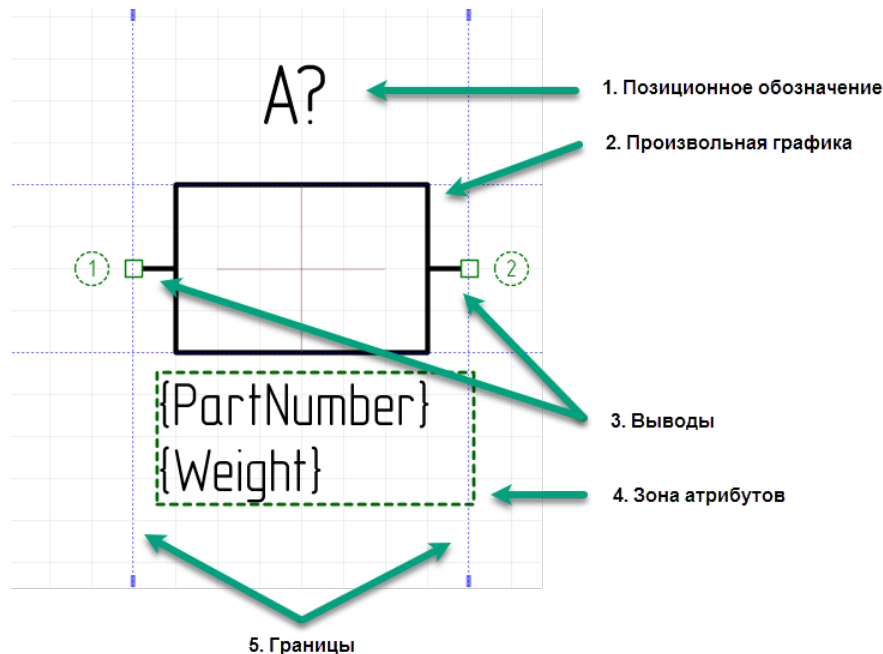
Рис. 161 Структурные элементы УГО
