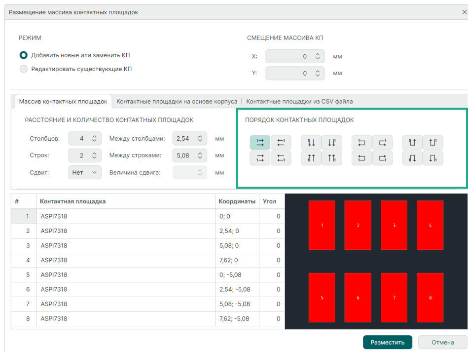
Рис. 89 Порядок нумерации контактных площадок
