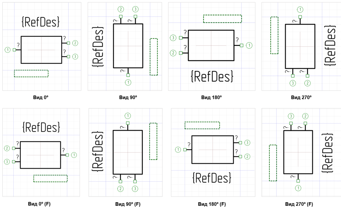
Рис. 237 Варианты ориентации УГО
