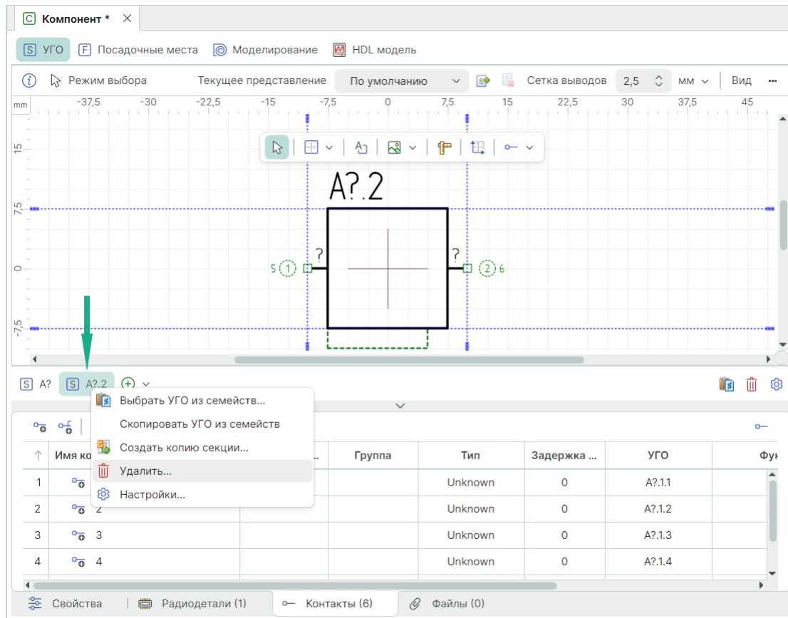
Рис. 206 Удаление секции
