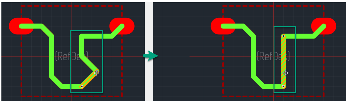
Рис. 123 Объединение сегментов
