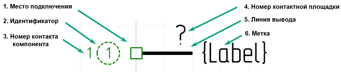
Рис. 162 Составляющие вывода
