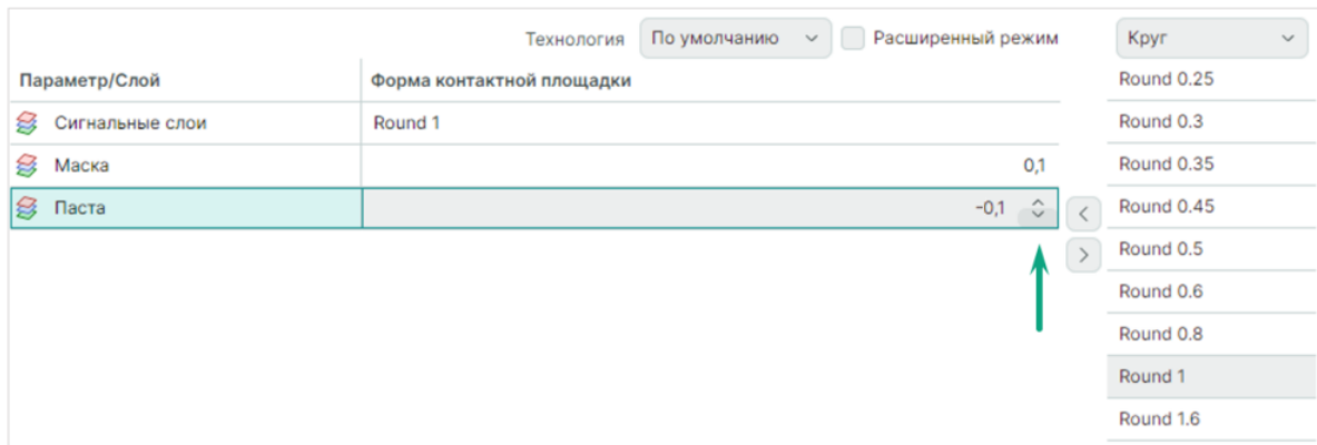
Рис. 46 Указание зазора и отступа для технологических слоев
