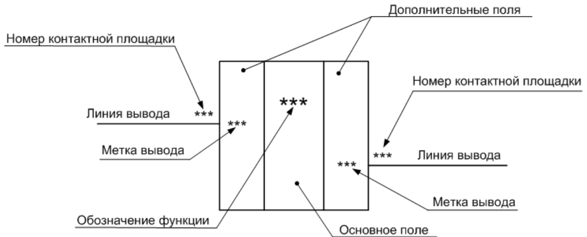
Рис. 216 Типовое УГО элемента цифровой техники
