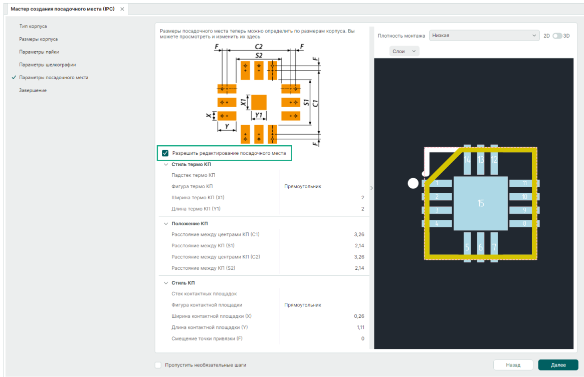
Рис. 143 Уточнение параметров посадочного места
