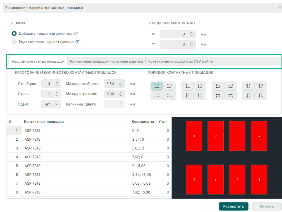
Рис. 88 Выбор варианта создания массива контактных площадок
