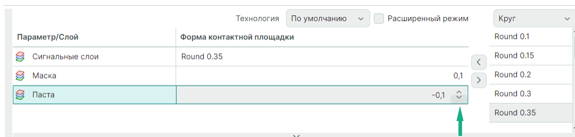
Рис. 60 Определение параметров пасты и маски для контактных площадок
