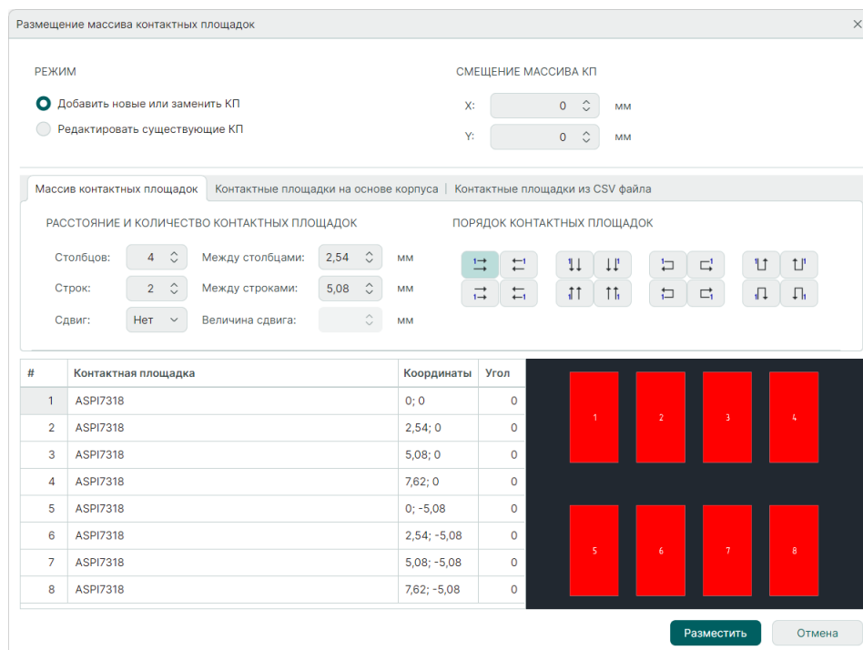
Рис. 87 Окно «Размещение массива контактных площадок»
