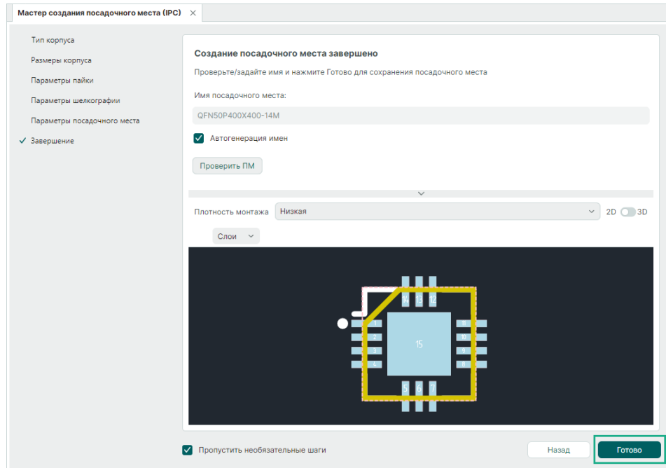
Рис. 146 Завершение создания посадочного места
