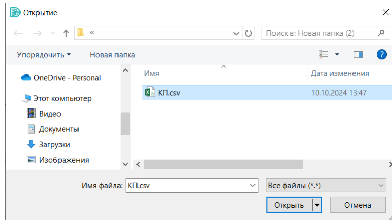
Рис. 102 Выбор csv-файла
