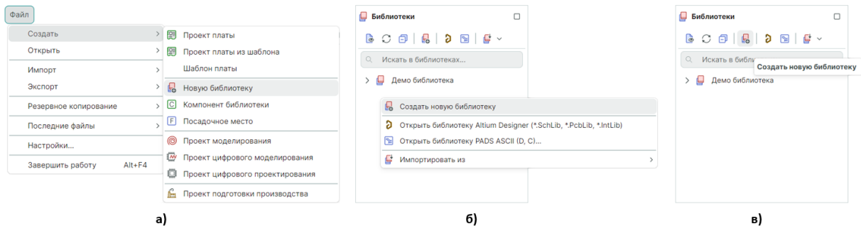
Рис. 3 Создание библиотеки
