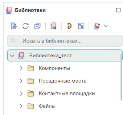
Рис. 5 Структура библиотеки
