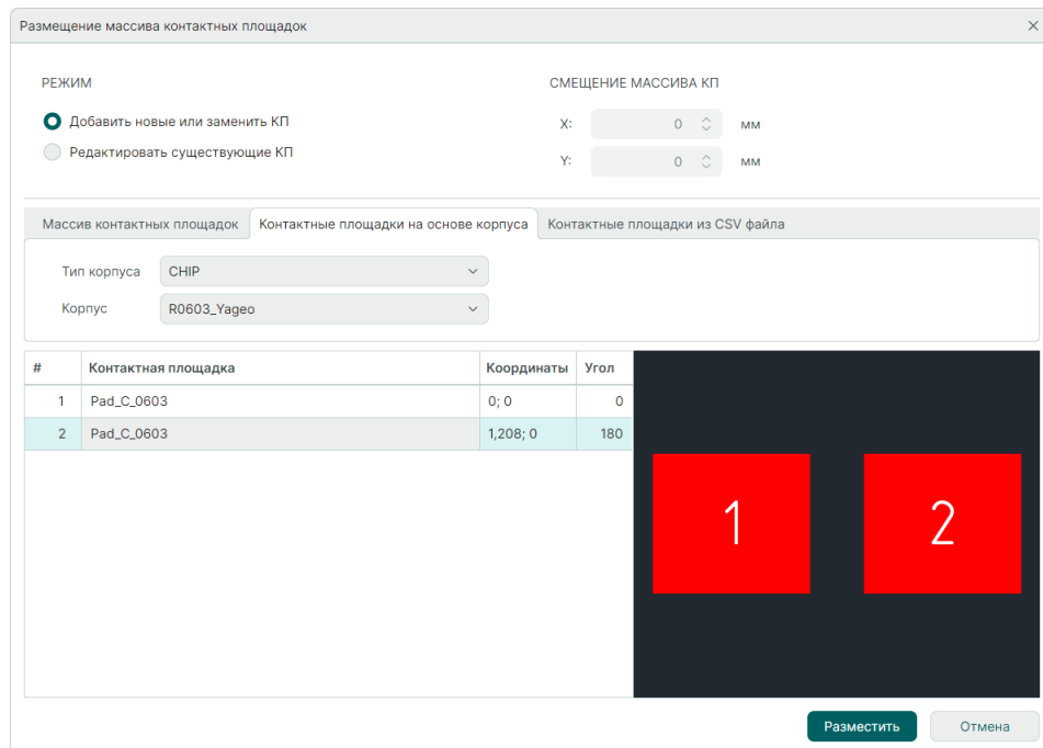
Рис. 98 Выбор корпуса
