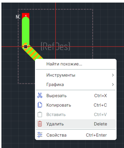
Рис. 127 Удаление сегмента
