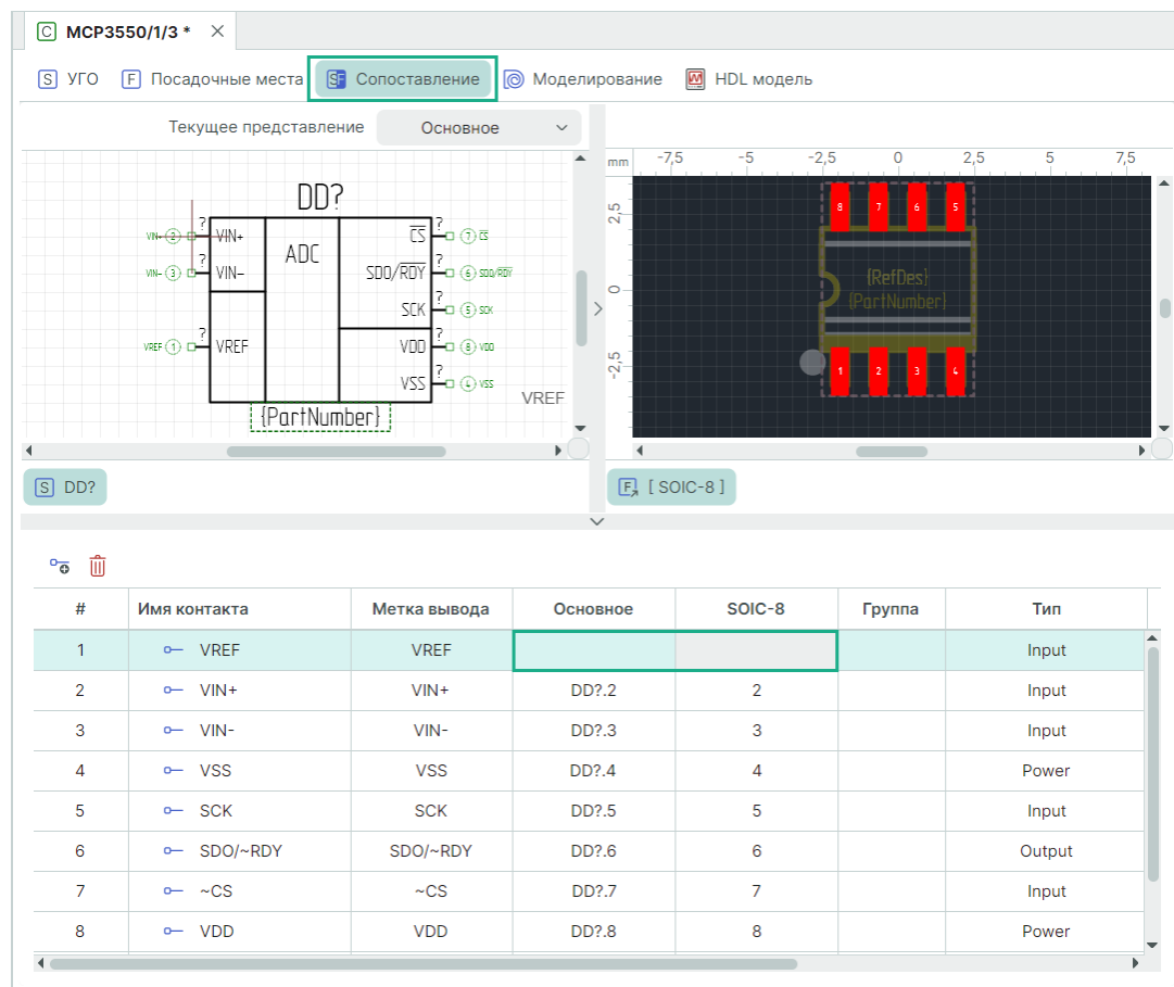
Рис. 264 Вкладка «Сопоставление»
