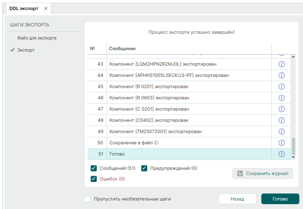
Рис. 34 Экспорт библиотеки
