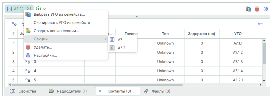
Рис. 203 Выбор секции
