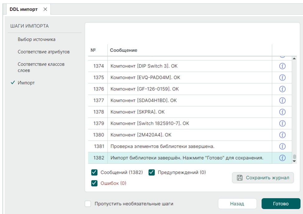
Рис. 28 Импорт библиотеки
