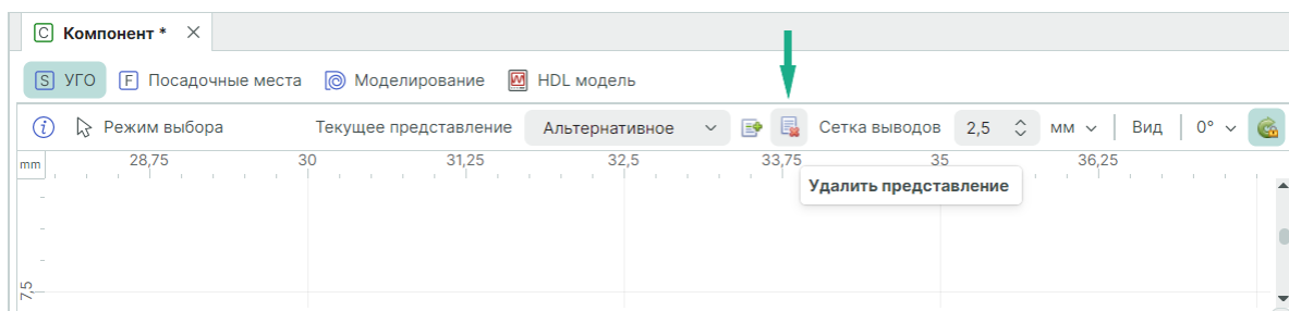
Рис. 234 Удаление представления
