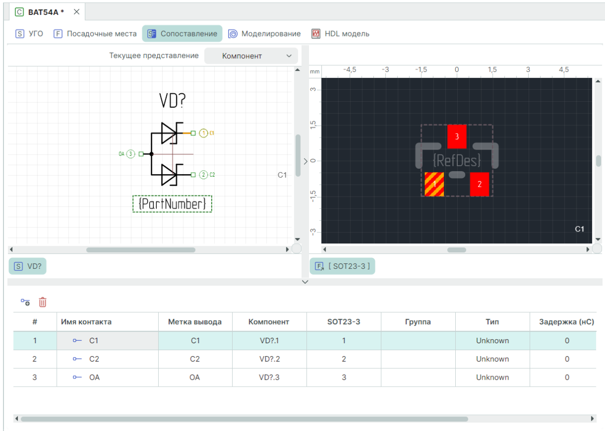
Рис. 244 Вкладка «Сопоставление»
