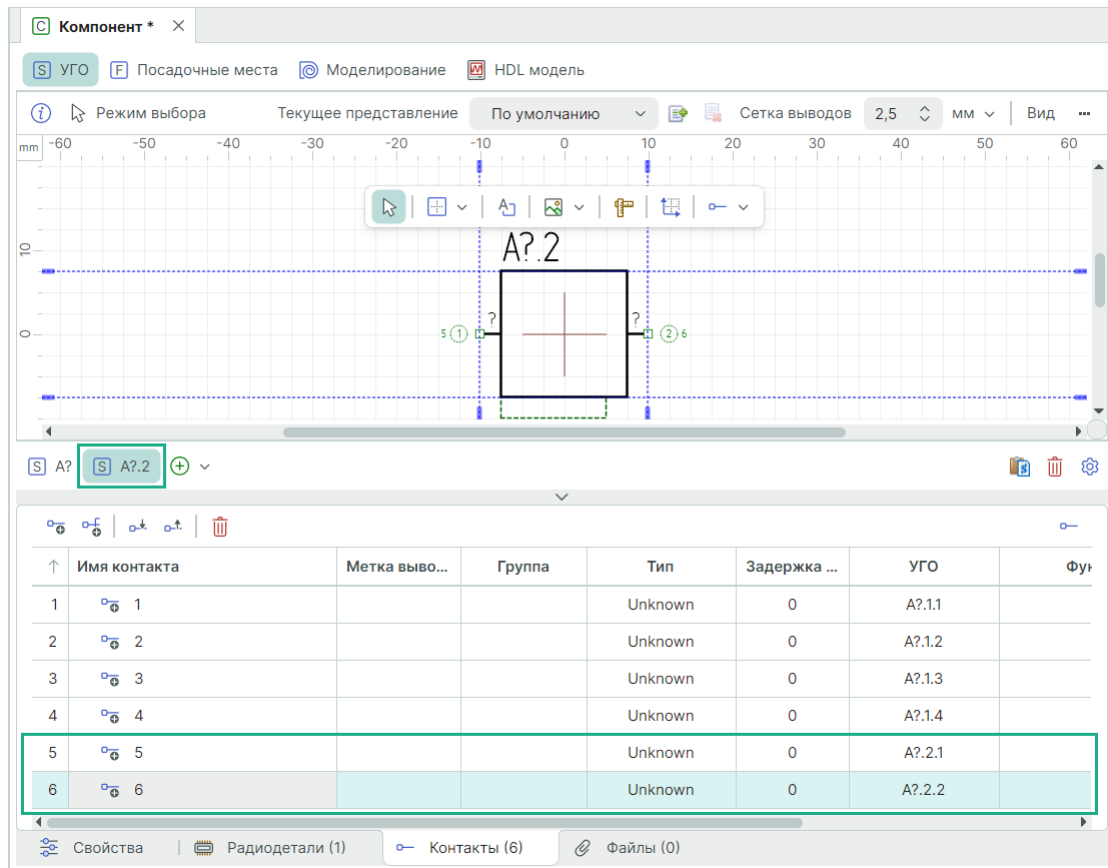
Рис. 205 Новая секция
