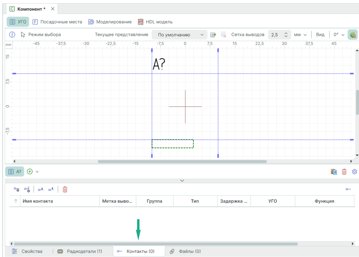
Рис. 241 Вкладка «Контакты»
