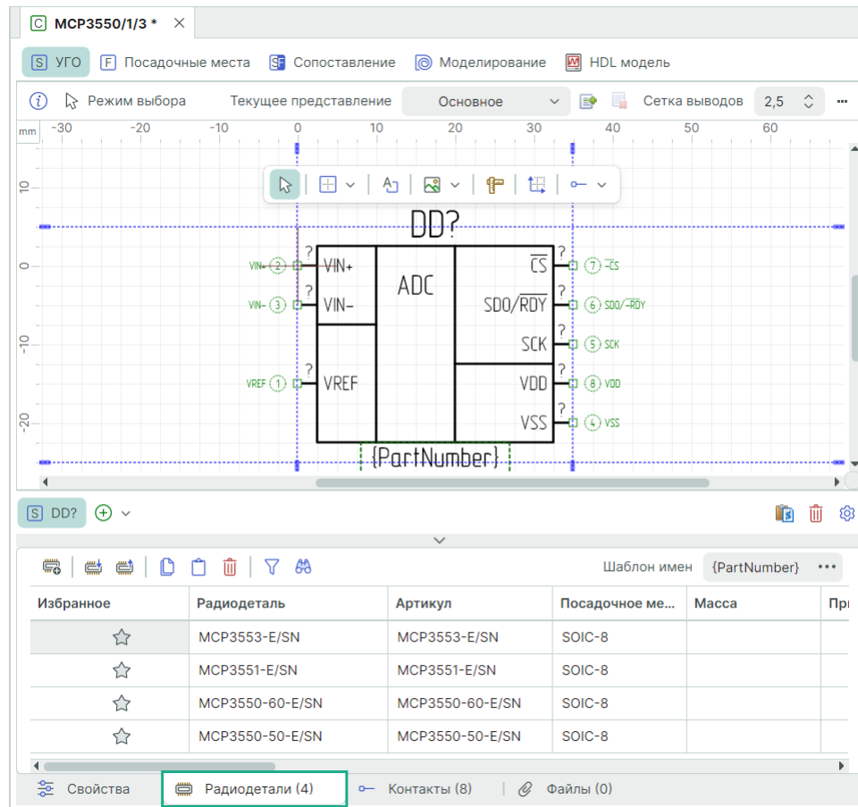
Рис. 294 Вкладка «Радиодетали»
