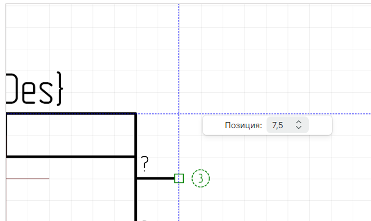
Рис. 171 Направляющая линия
