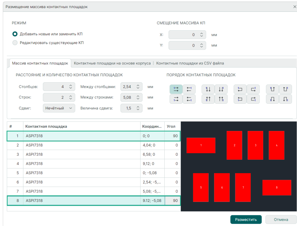
Рис. 95 Индивидуальные координаты и углы поворота контактных площадок
