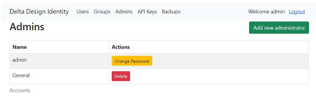
Рис. 82 Страница «Admins» (Администраторы)
