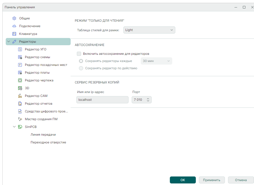
Рис. 77 Доступные настройки службы резервного копирования
