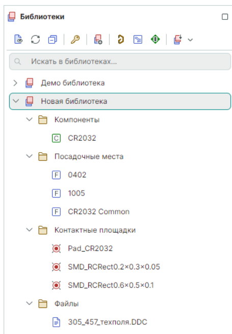
Рис. 89 Панель «Библиотеки»
