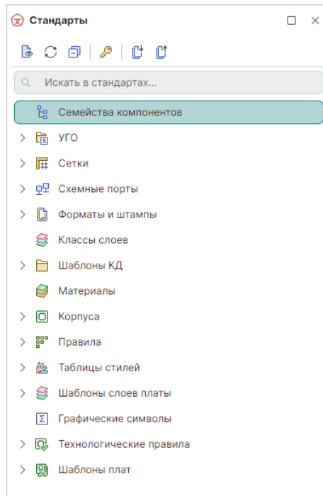
Рис. 88 Панель «Стандарты»
