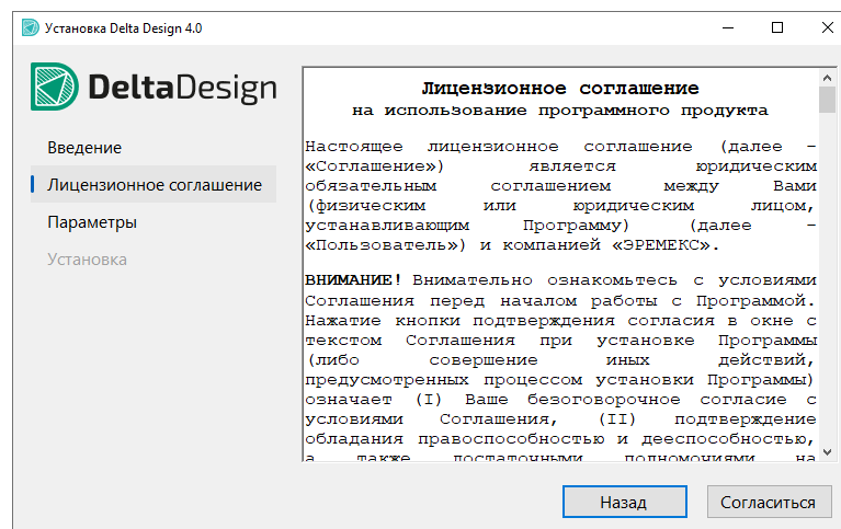
Рис. 2 Лицензионное соглашение
