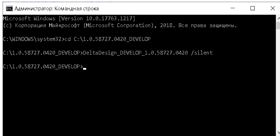
Рис. 23 Запуск тихой установки
