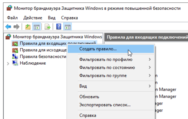
Рис. 66 Создание нового правила для работы брандмауэра
