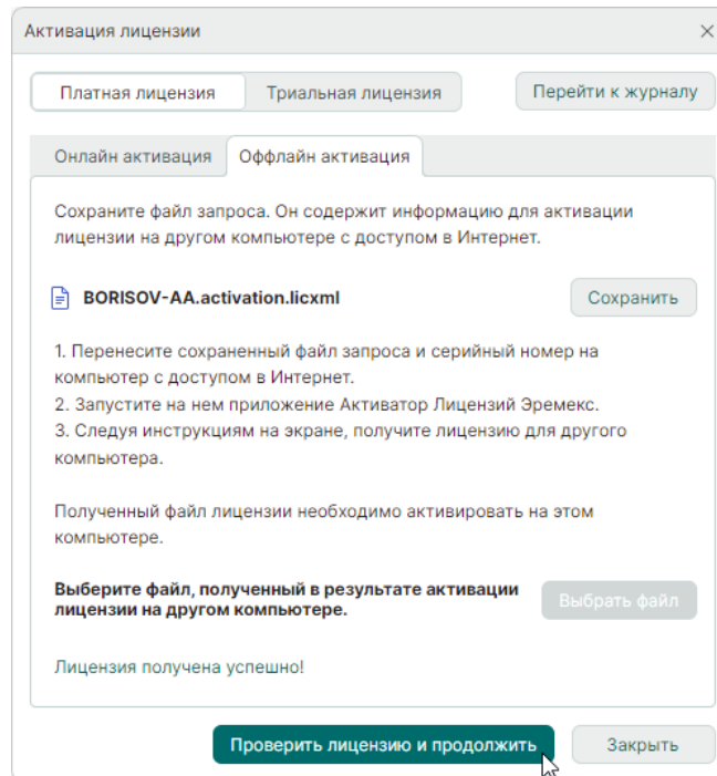
Рис. 60 Завершение активации
