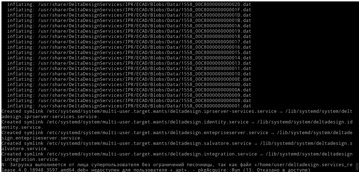
Рис. 42 Завершение установки
