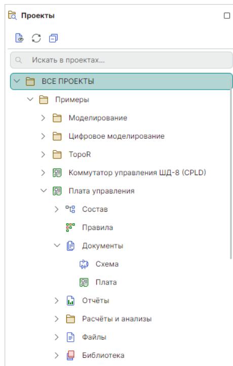
Рис. 90 Панель «Проекты»
