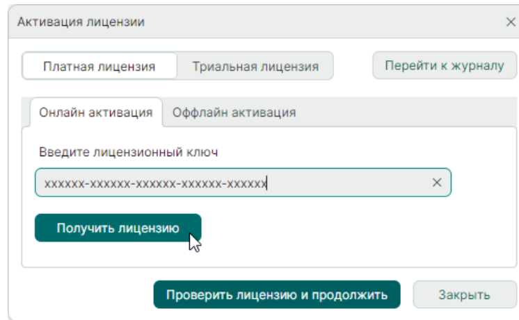
Рис. 49 Получение лицензии
