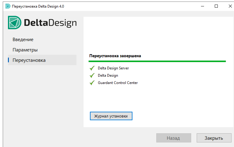
Рис. 9 Завершение переустановки
