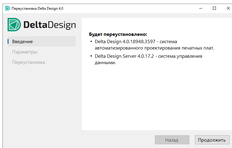
Рис. 6 Переустановка системы
