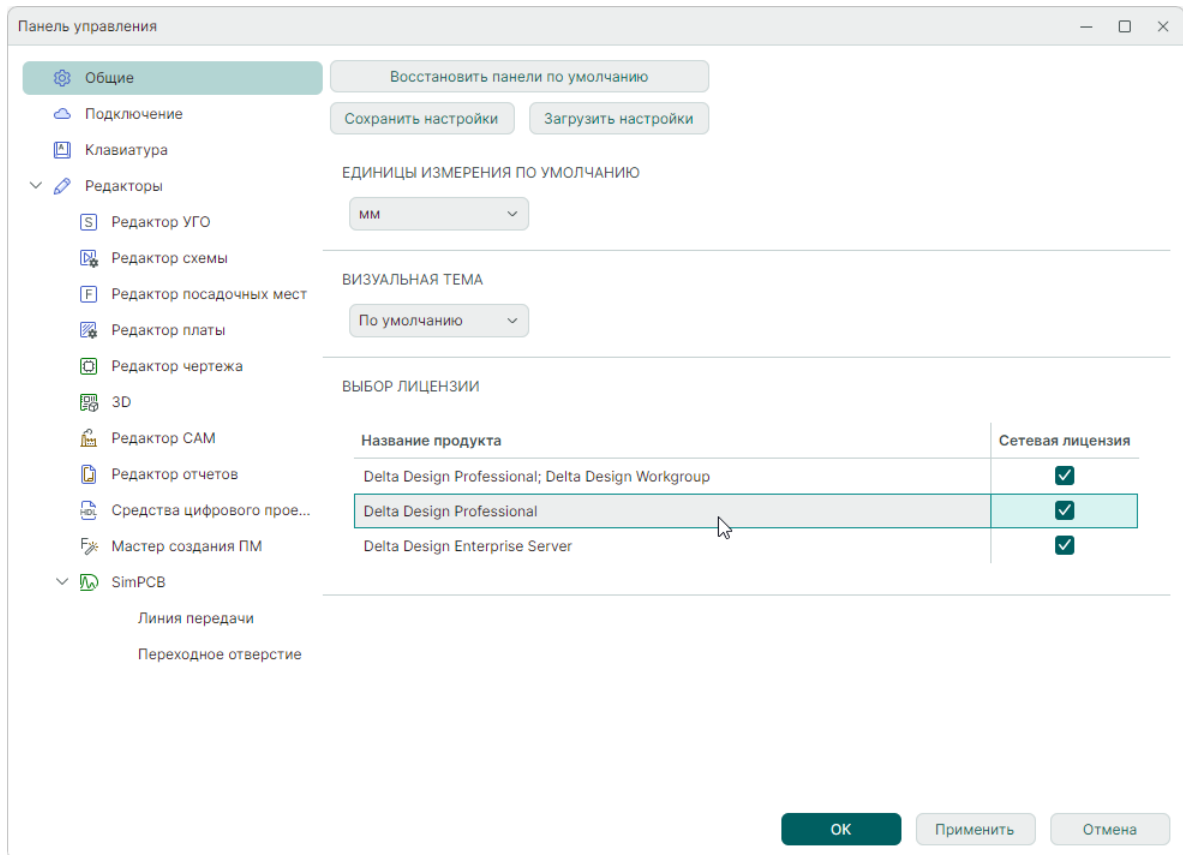
Рис. 63 Доступные лицензии
