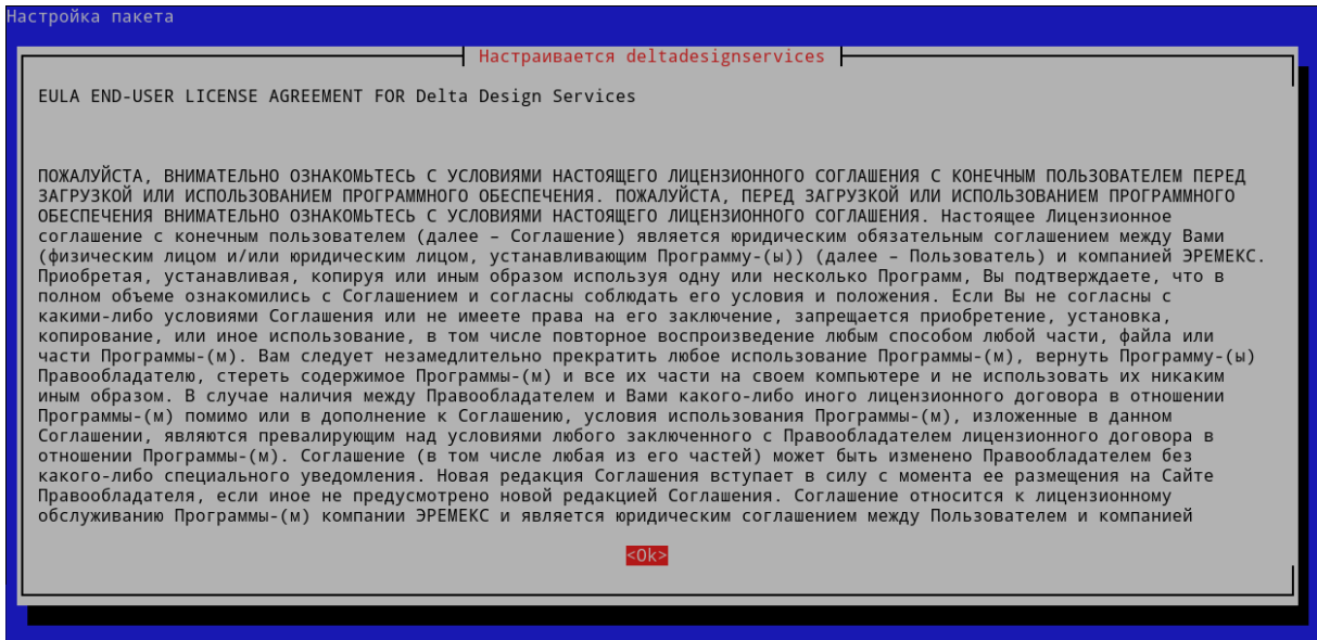
Рис. 34 Лицензионное соглашение
