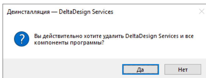
Рис. 46 Подтверждение удаления
