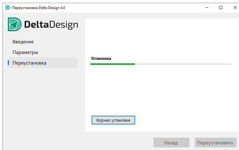
Рис. 8 Выполнение переустановки
