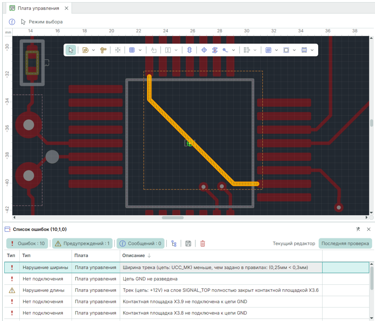
Рис. 534 Переход к нарушению в редакторе плат
