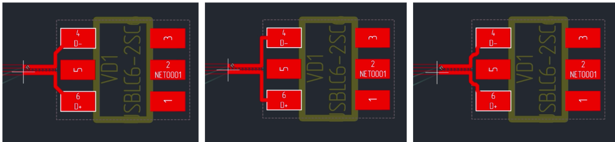
Рис. 327 Варианты симметричного соединения с КП
