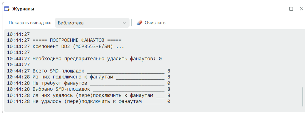
Рис. 305 Итоговая информация по построенным фанатам
