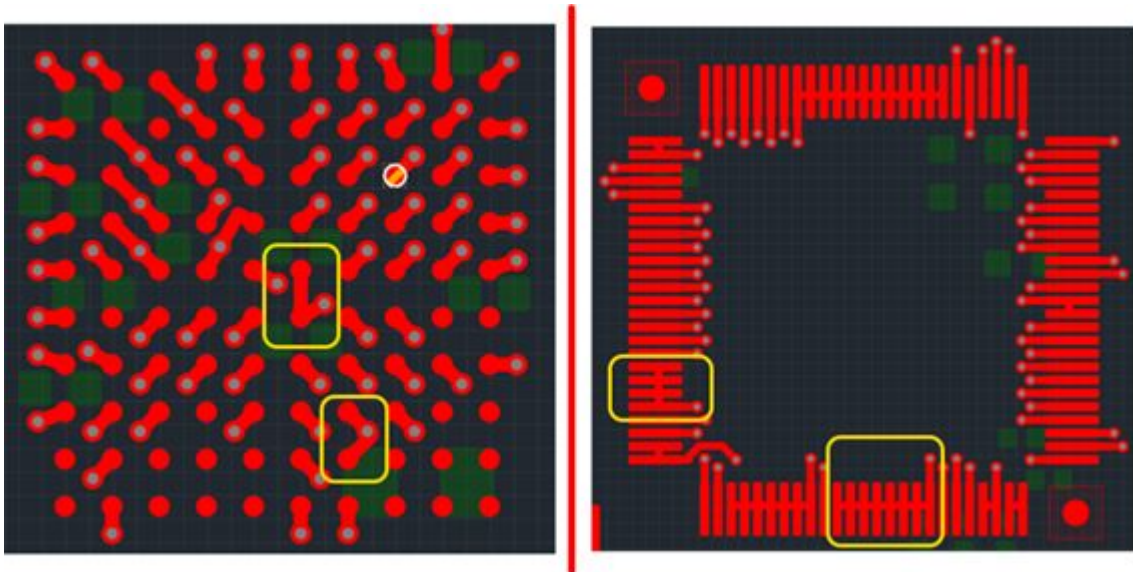
Рис. 314 Пример построения общих фанатов
