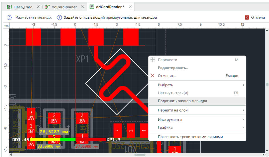
Рис. 382 Вызов инструмента «Подогнать размер меандра»
