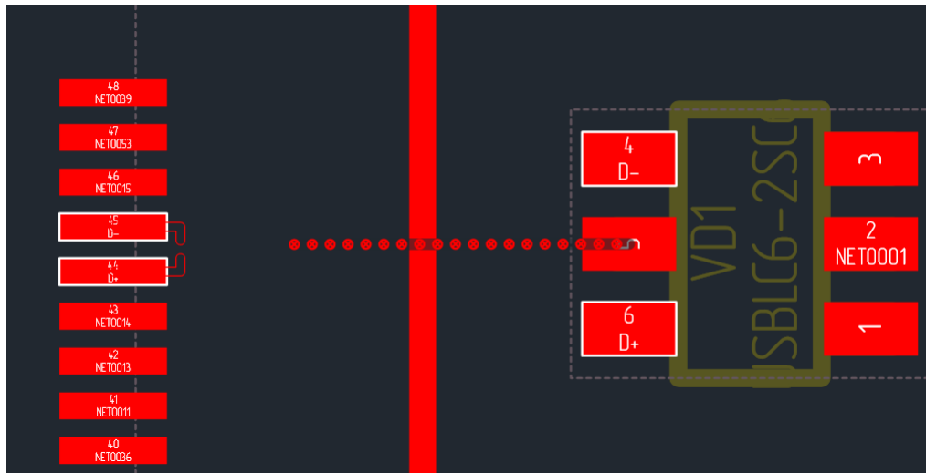
Рис. 331 Отображение некорректного варианта трассировки диффпары
