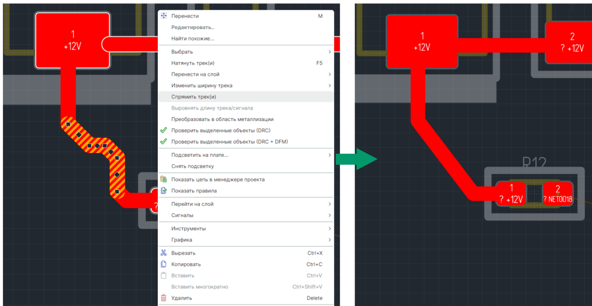
Рис. 214 Спрямление участка трека
