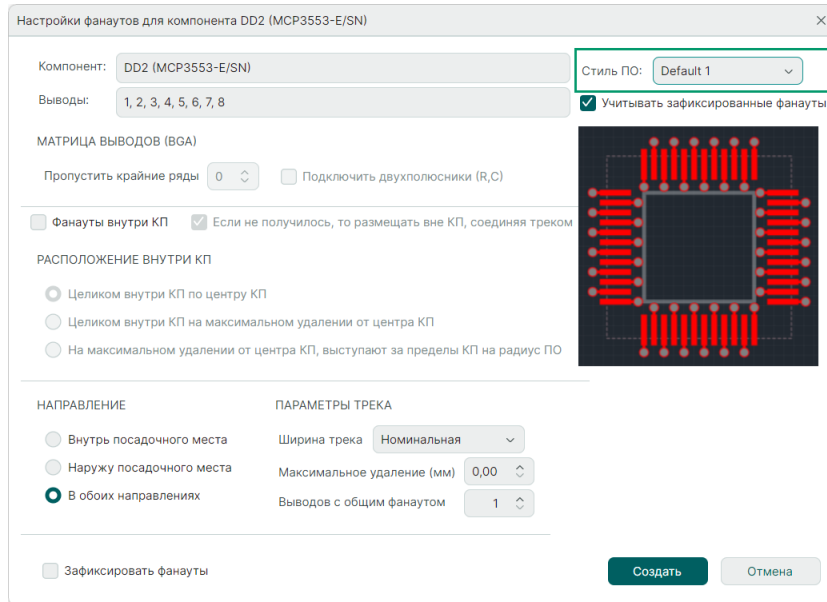
Рис. 299 Выбор стиля переходного отверстия
