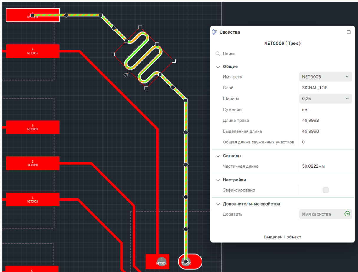
Рис. 385 Выравнивание задержки (длины) сигнала по заданному значению
