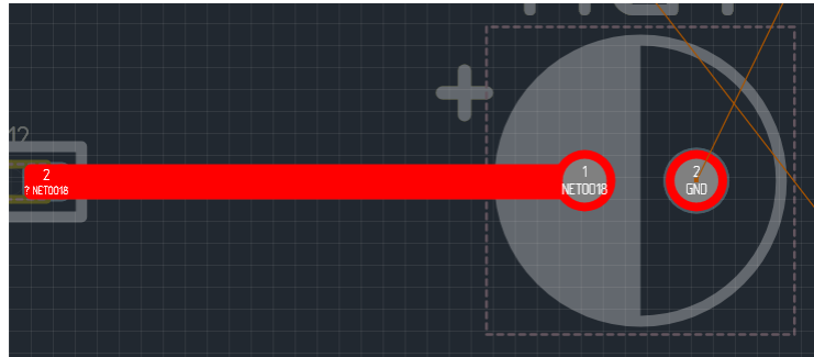
Рис. 267 Результат спрямления трека
