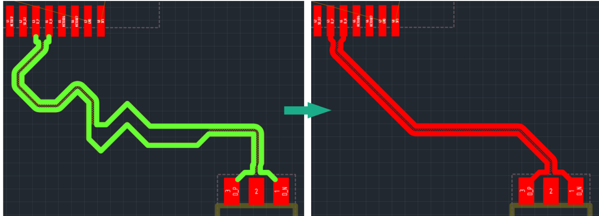
Рис. 347 Натяжение диффпары
