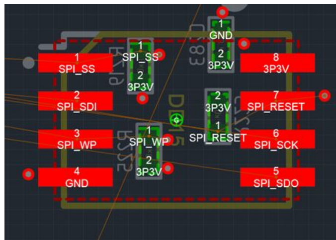
Рис. 196 Отображение номера контактной площадки и имени цепи
