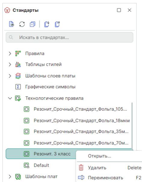
Рис. 519 Доступные действия с созданными шаблонами правил
