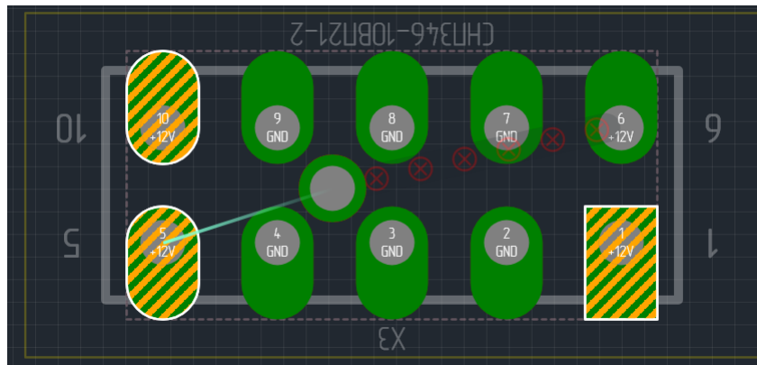
Рис. 220 Место, запрещенное для размещения перехода
