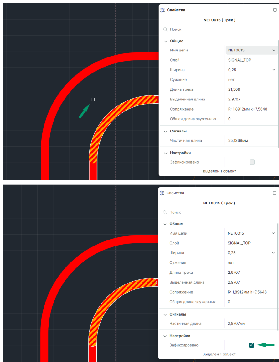
Рис. 293 Применение фиксации области трека
