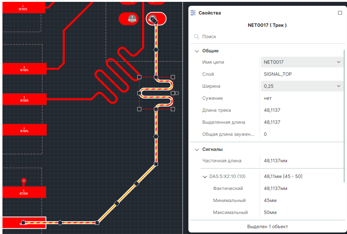
Рис. 392 Выравнивание длины сигнала в режиме «По другому сигналу»
