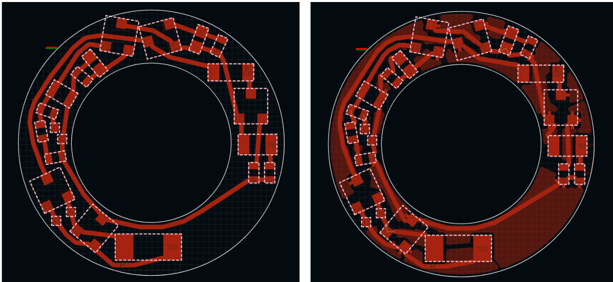
Рис. 406 Вид проводников до преобразования (слева) и после преобразования (справа) в область металлизации
