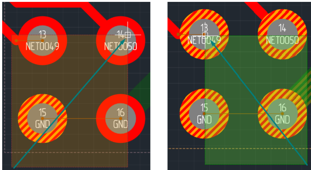
Рис. 86 Вариативность инструмента «Выбрать» от направления движения курсора при создании области выбора
