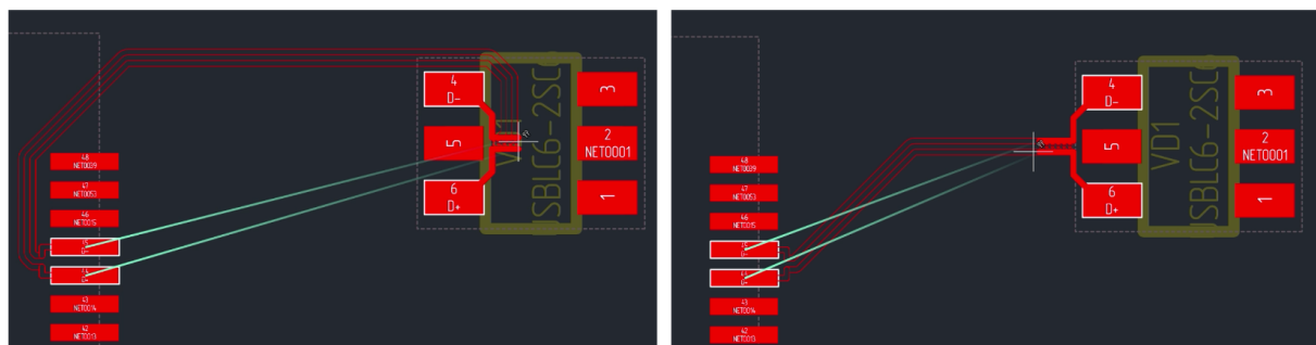
Рис. 330 Варианты соединения диффпары со стартовой парой контактных площадок
