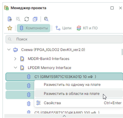
Рис. 128 Выбор группы в рамках
