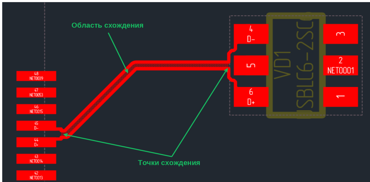
Рис. 329 Точки схождения и область схождения диффпары
