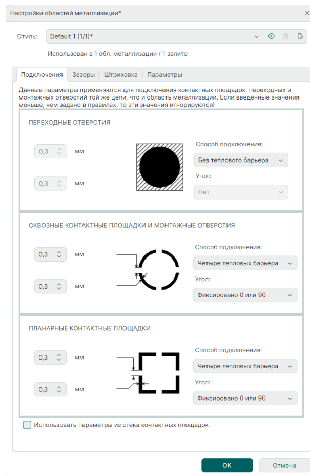
Рис. 440 Окно «Настройки областей металлизации»
