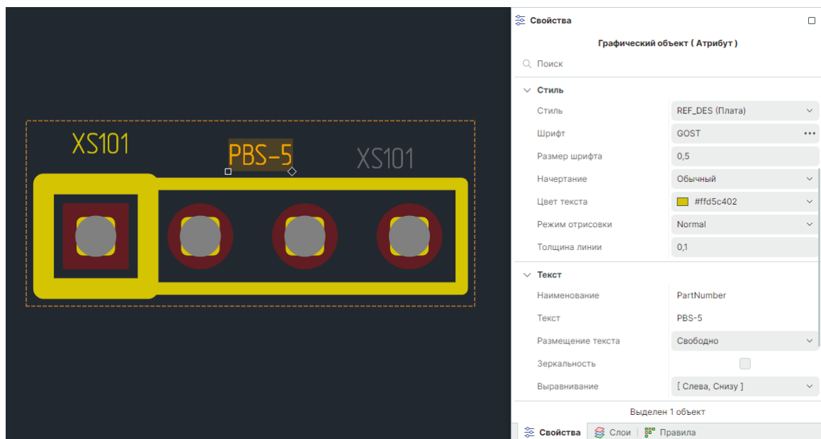
Рис. 154 Изменение свойств атрибута как графического объекта
