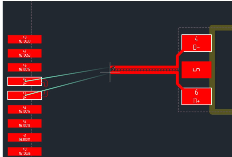
Рис. 333 Возможный вид прокладываемого участка диффпары
