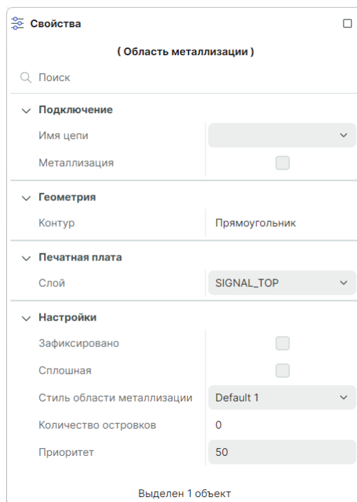
Рис. 433 Свойства области металлизации
