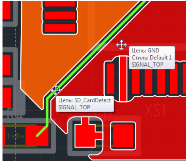
Рис. 458 Пример разделения области металлизации трек
