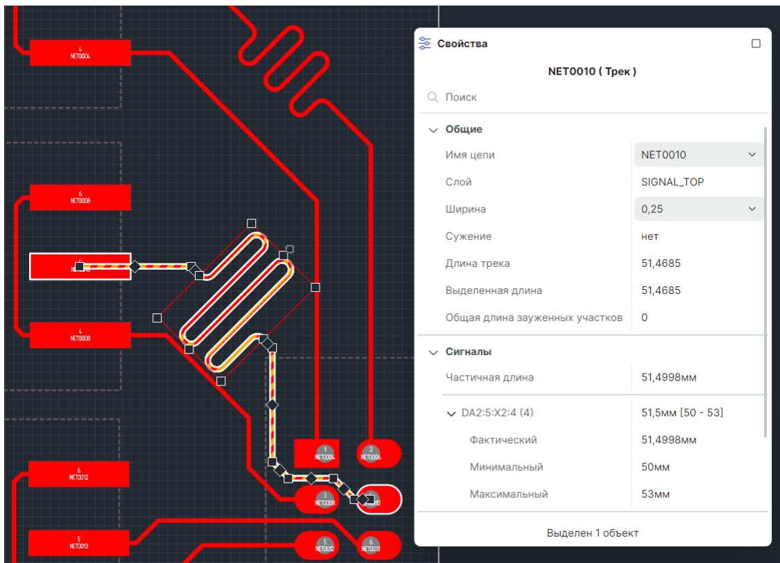
Рис. 389 Выравнивание длины сигнала в режиме «Автоматически»
