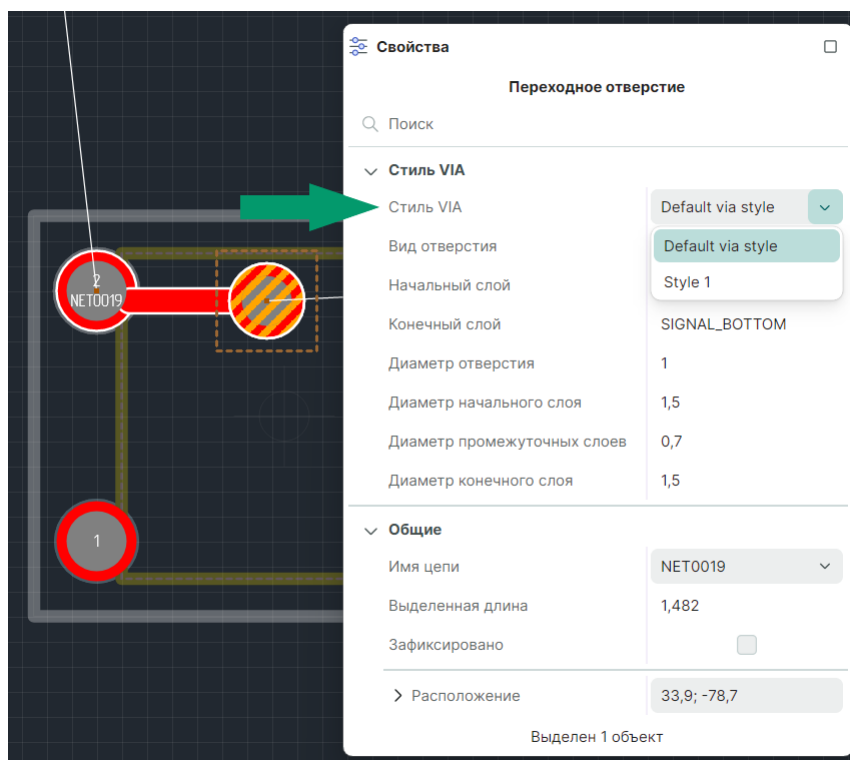
Рис. 221 Изменение стиля переходного отверстия
