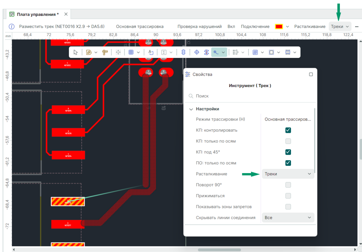
Рис. 237 Размещение трека в режиме расталкивания
