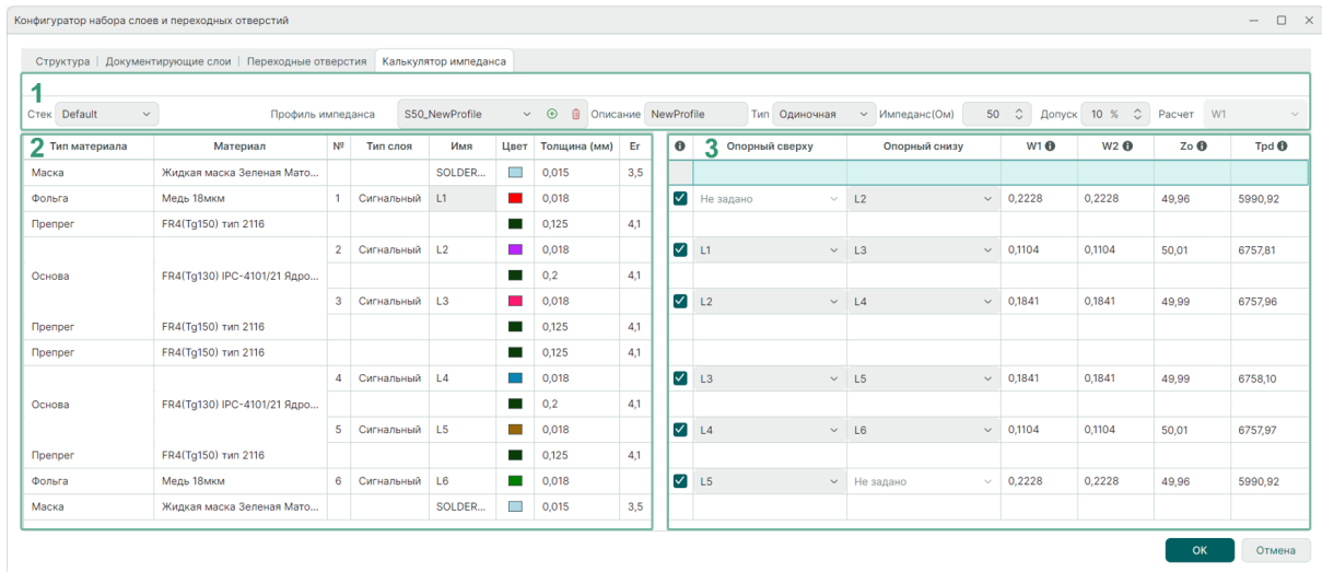
Рис. 38 Профиль импеданса
