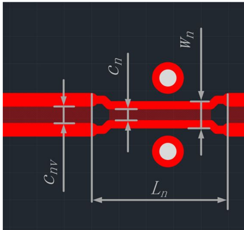
Рис. 323 Параметры диффпар
