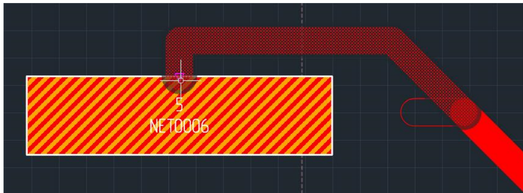
Рис. 262 Вариант нового подключения к контактной площадке
