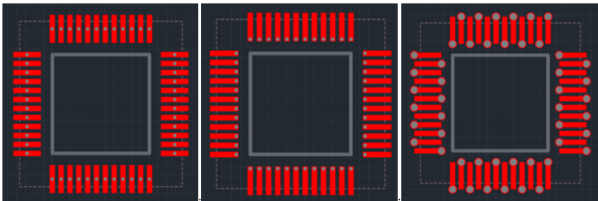
Рис. 309 Различные варианты расположения фанатов относительно КП
