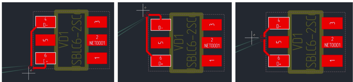
Рис. 328 Варианты несимметричного соединения с КП
