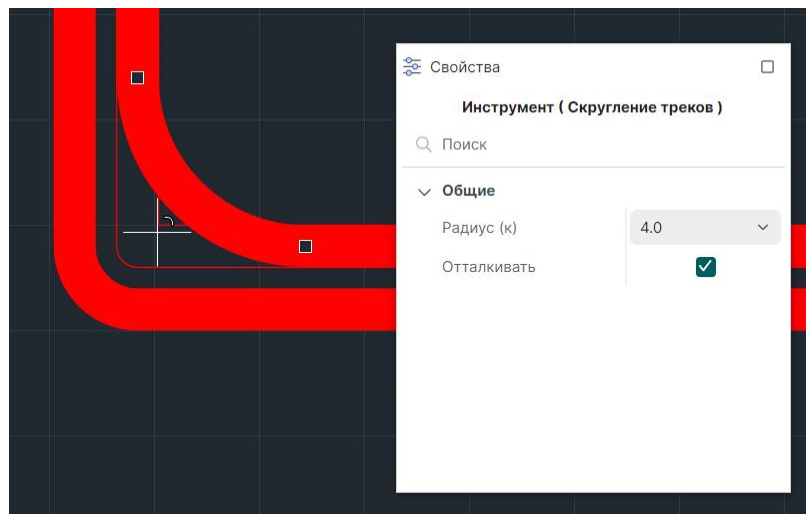
Рис. 346 Скругление угла на "расстегнутом" участке диффпары
