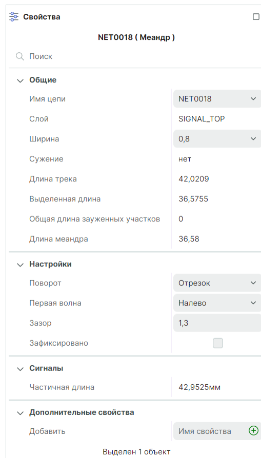
Рис. 271 Свойства меандра
